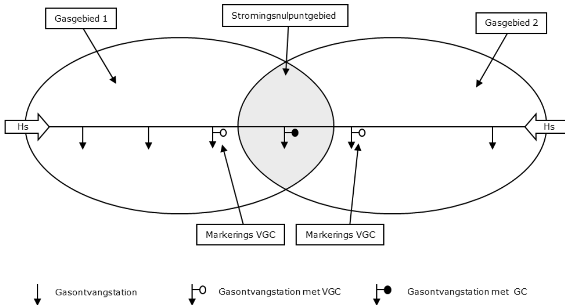
Figuur 2: Stromingsnulpuntgebied
