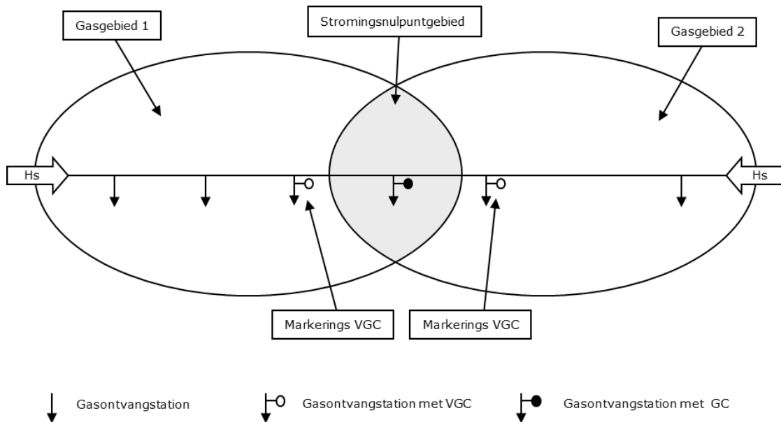
Figuur 2: Stromingsnulpuntgebied
