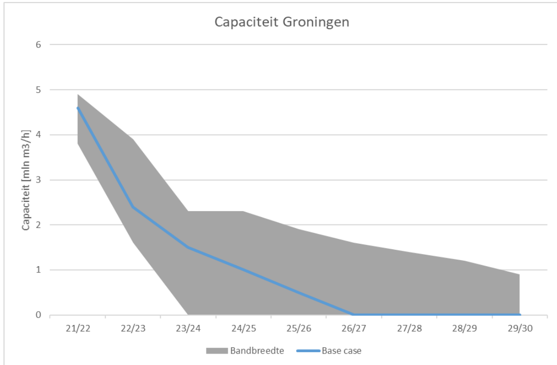
Figuur 9: Benodigde Groningencapaciteit tot gasjaar 2029/2030, inclusief gevoeligheidsanalyse
