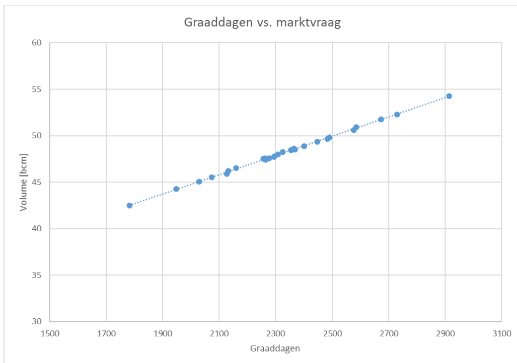
Figuur 4: Benodigde L-gasvraag in gasjaar 2020/2021 die vanuit Nederland moet worden beleverd op basis van de laatste 30 temperatuurprofielen
